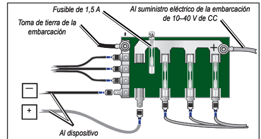
Ejemplo de bloque de fusibles
